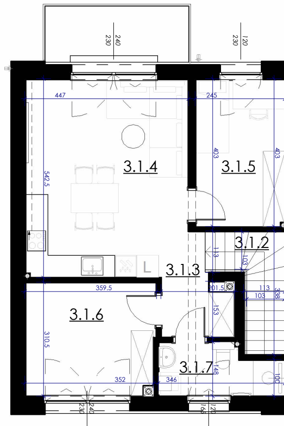
RZUT PIĘTRA
