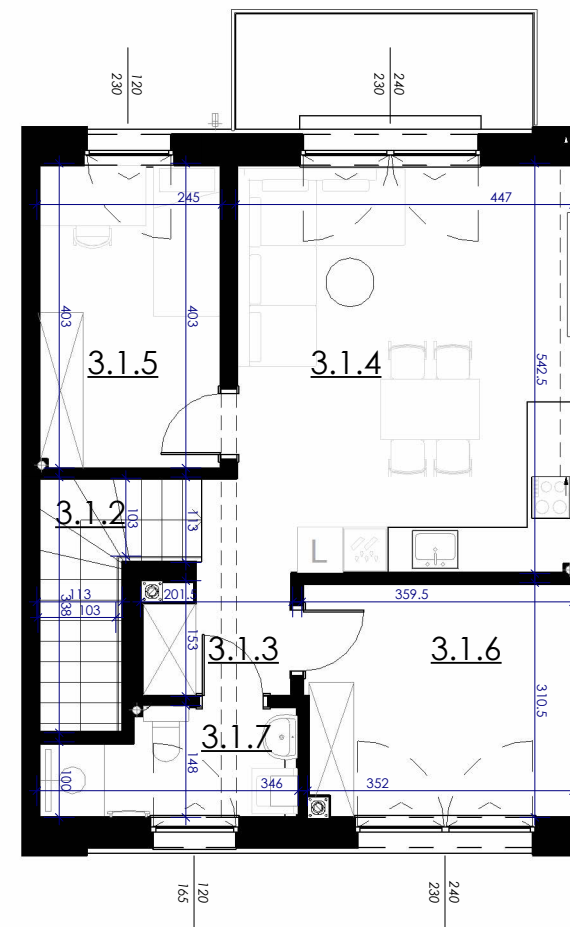
RZUT PIĘTRA
