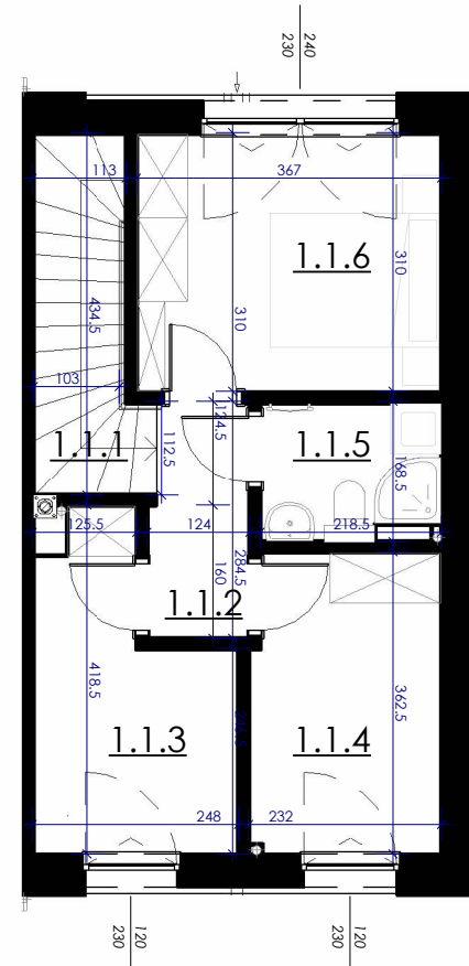
RZUT PIĘTRA
