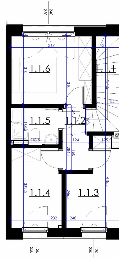
RZUT PIĘTRA
