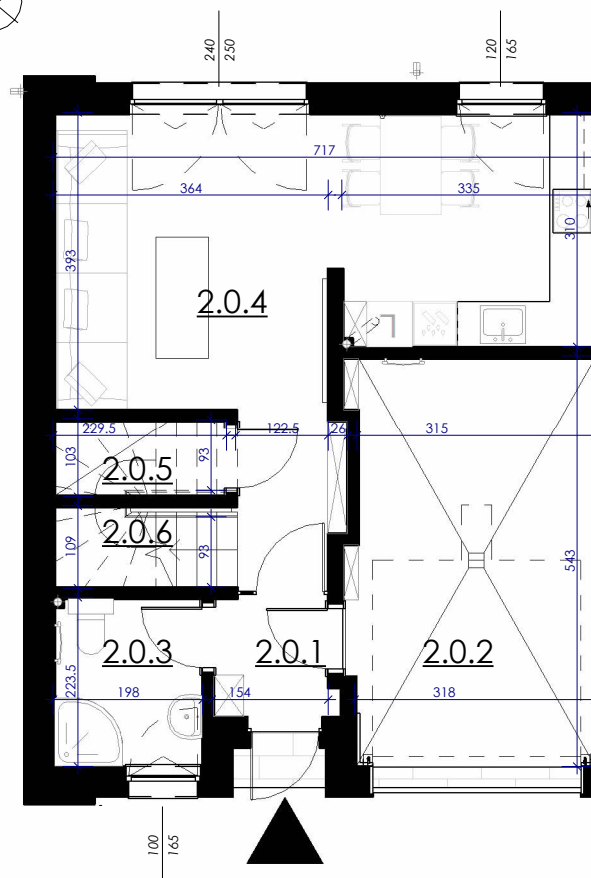
RZUT PARTERU
