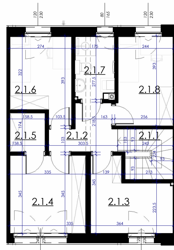
RZUT PIĘTRA
