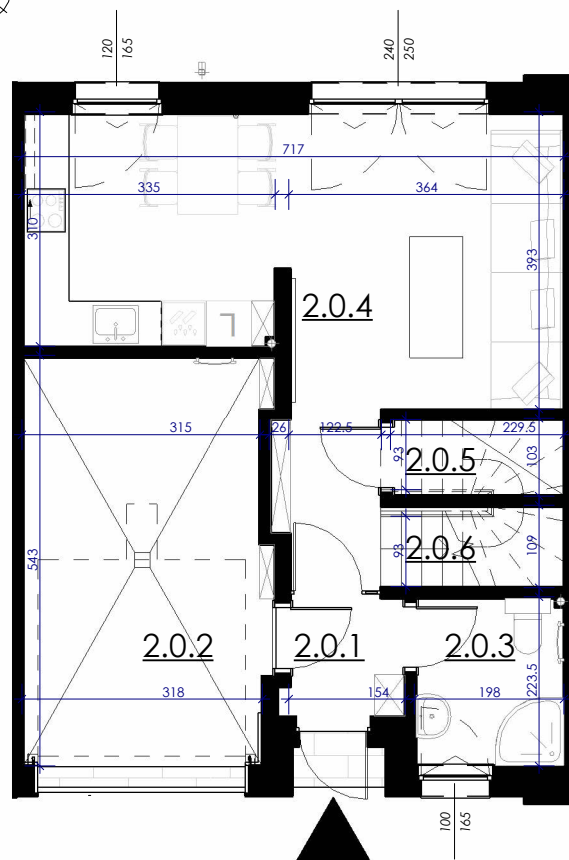
RZUT PARTERU
