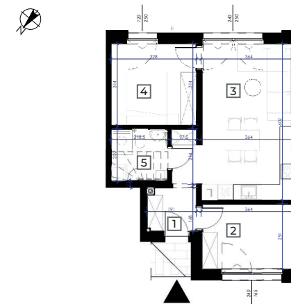
Rzut apartamentu
