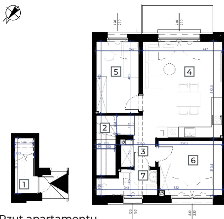
Rzut apartamentu
