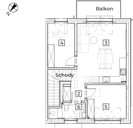
Rzut apartamentu
